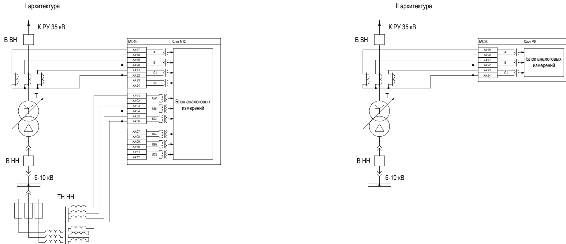
Рисунок В.1 – Подключение аналоговых цепей трансформаторов тока и напряжения двухобмоточного трансформатора 35 кВ к устройству
