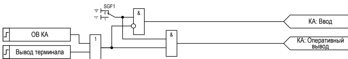
Рисунок 2.26 – Логика управления режимами функционального блока «КА»
