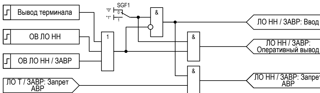
Рисунок 2.19 – Функциональная схема логики запрета АВР
