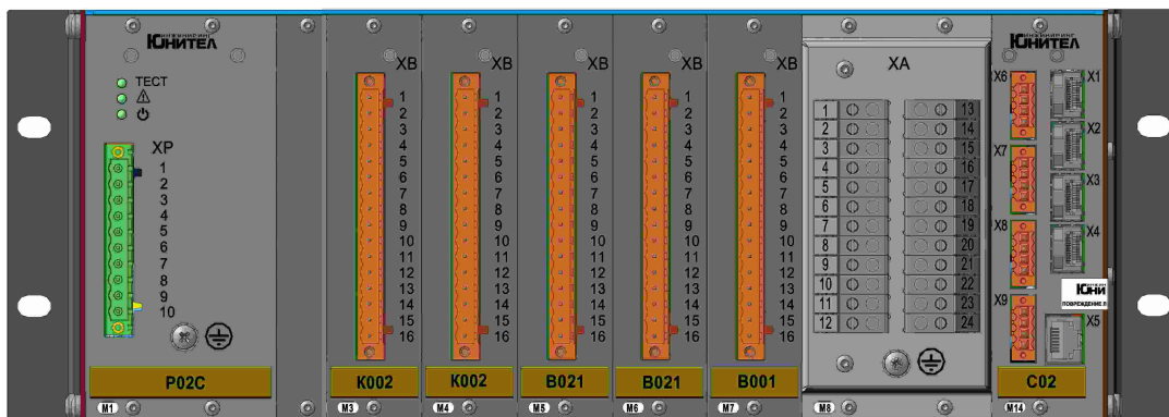
Рисунок 1.2 – Вид устройства «ЮНИТ-М314-Т2» с размещением блоков по слотам (исполнение для II архитектуры)
